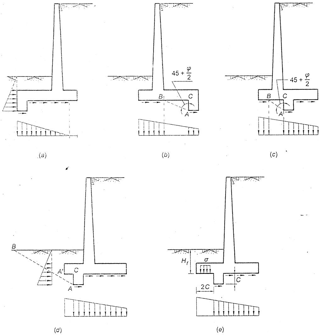
Schemi utilizzati per la redazione degli Abachi C3-C6.
