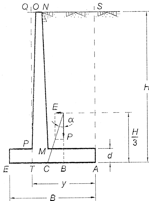
Predimensionamento di un muro a mensola.
